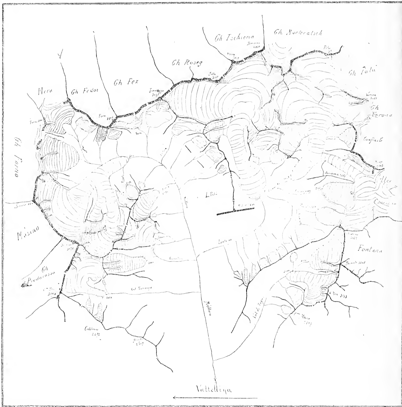
Fig. 3. — Ricostruzione dei ghiacciai di Val Malenco nello stadio Daun .
